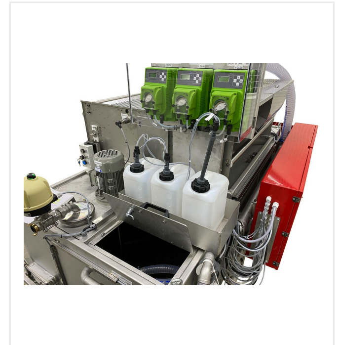
Vorratsbehälter und Dosierstation für Flockungsmittel optional Reinigungsmittel etc.
