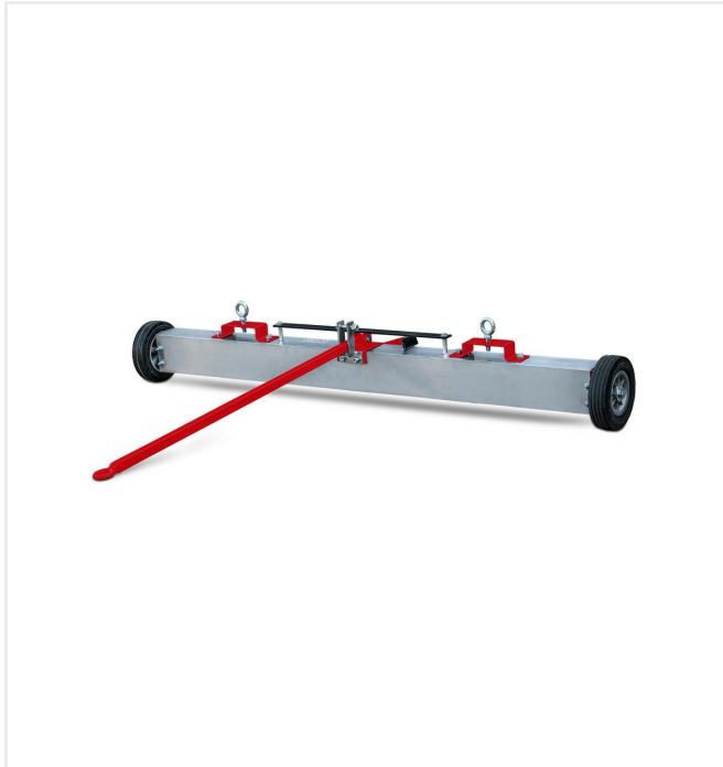
Magnetleiste ML1500
