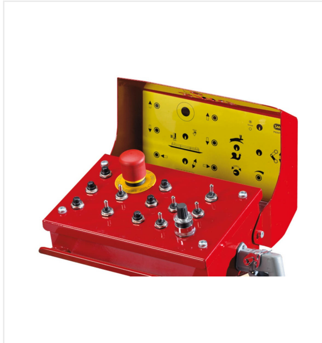
Steuerpanel, beidseitig angebracht, sämtliche Bedienfunktionen inkl. Kurvensteuerung integriert
