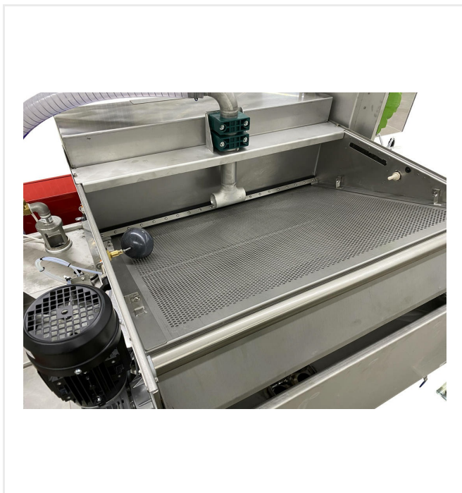
Filtro de banda con tamiz filtrante resistente al desgarrado (120 \mu m) que incluye recipiente colector con interruptor flotante
