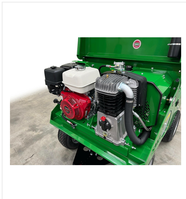
Chłodzony powietrzem silnik spalinowy do napędzania pomp i kompresorów (możliwość wyboru silnika elektrycznego)
