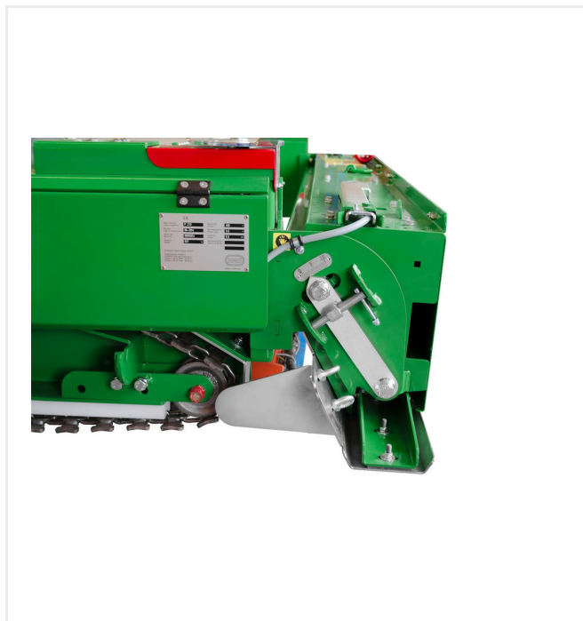
Регулировка угла наклона разравнивателя, ограничители по бокам для однородной и бесшовной укладки
