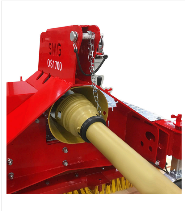
Zapfwelle mit Heckdreipunktaufnahme, Antrieb über Zapfwelle
