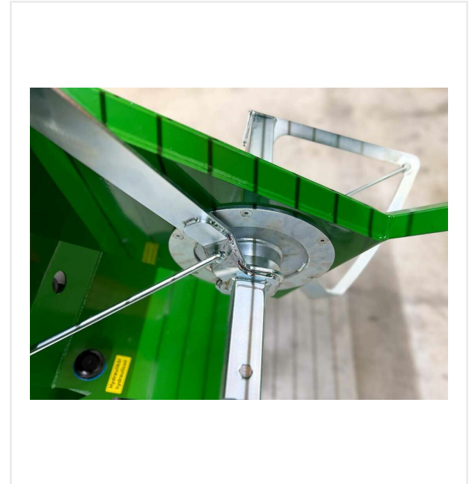
Mischwerkzeug im Mischkopf integriert und hydraulisch anzuheben
