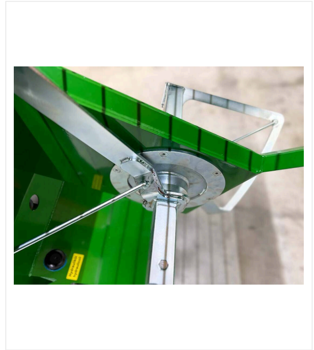
Mischwerkzeug im Mischkopf integriert und hydraulisch anzuheben
