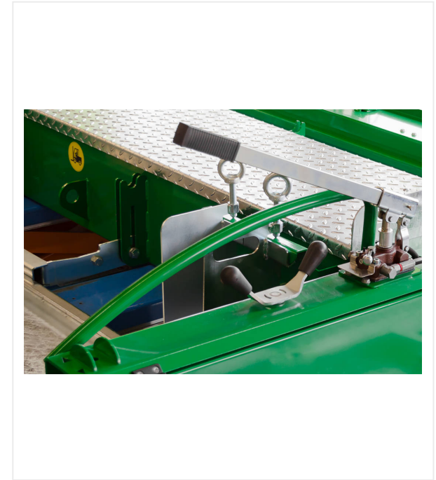
Handpumpe für manuelles Ein-/Ausfahren des Transport-Fahrwerkes.
