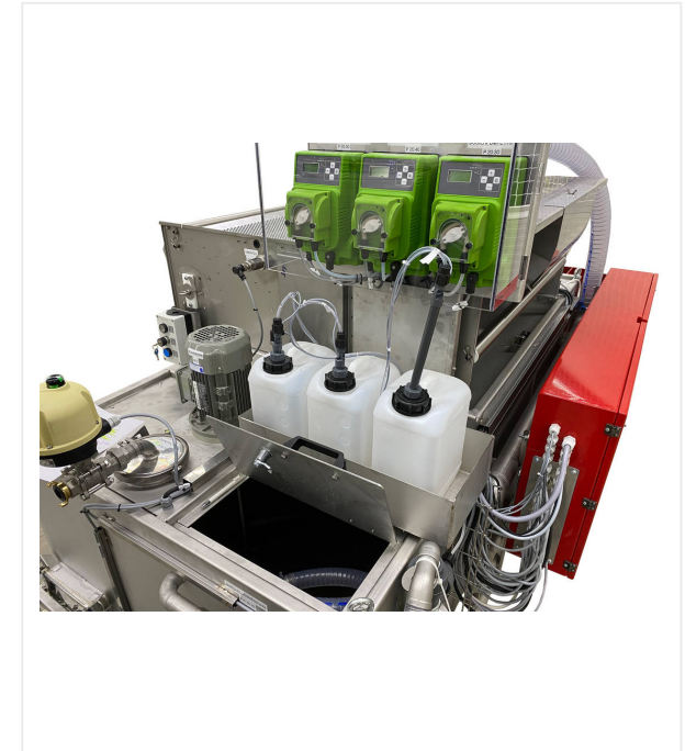
Tanque de almacenamiento y estación de dosificación para floclulantes, opcionalmente agentes de limpieza, etc.
