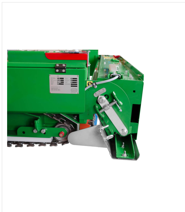
Réglage de l'inclinaison de la règle à araser, limiteur de matériau latéral pour une pose homogène.
