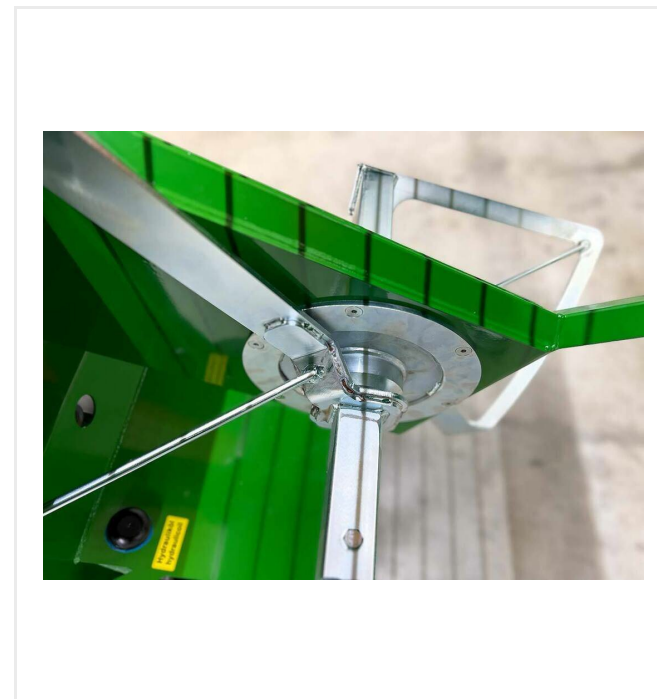
Outil de mélange intégré dans la tête de mélange et relevable
