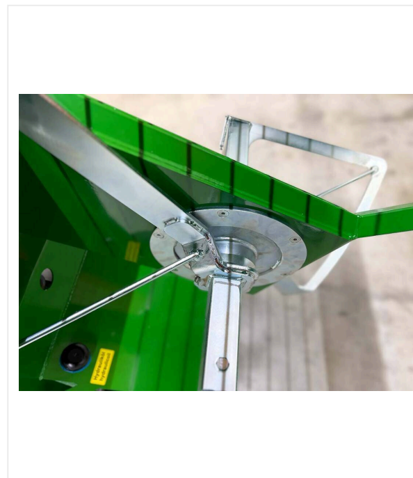
Narzędzie mieszające zintegrowane w głowicy mieszalnika i podnoszone hydraulicznie
