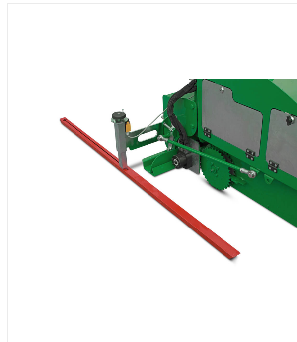
Opcjonalne szyna czułka do próbkowania podłoża
