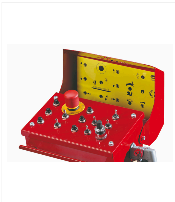
Centralny panel sterowania, przechylny
