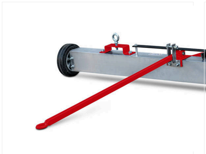
Listwa magnetyczna ML1500
