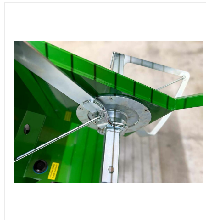
Смесительный инструмент, встроенный в смесительную головку, с гидравлическим подъемом
